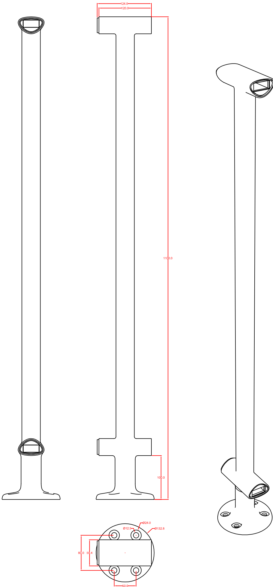
COLUMNA FIJA V1100
